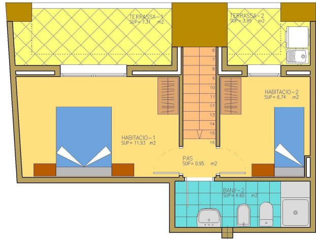
Plta. Sotacoberta Sup. Útil: 24.22m 2
