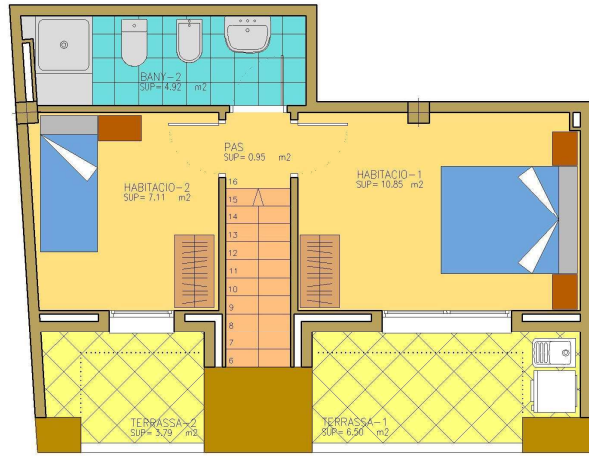
Plta. Sotacoberta Sup. Útil: 23.83m 2
